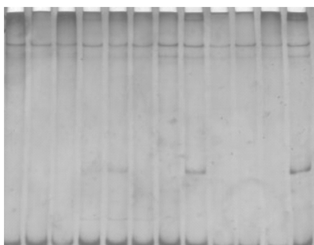
BCG H37RV3/86 85/91128/92175/94 3892 3893 3915 3916 3917 3012
